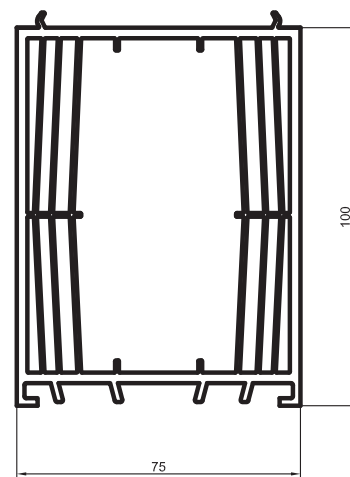
Toktoldó profil penta plus 100mm - 2586
