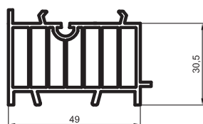
Alátét profil penta plus 2562
