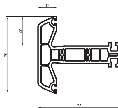
Szűk osztó penta plus 2532
