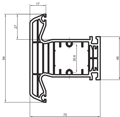
Széles osztó penta plus 2534
