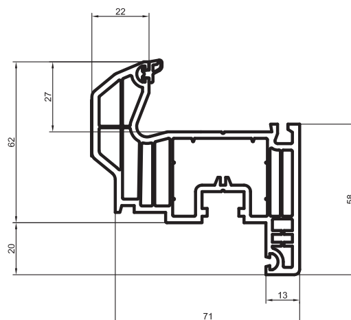
Ablak szárny penta plus 2528
