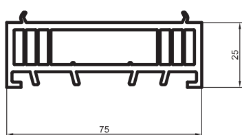
Toktoldó profil penta plus 25mm - 2584
