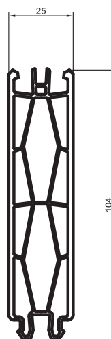
Ajtó betét lamella 2172
