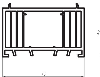
Toktoldó profil penta plus 45mm - 2585
