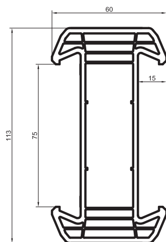
Összekötő I profil penta plus 2577
