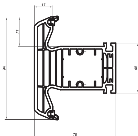
Széles osztó penta plus 2535
