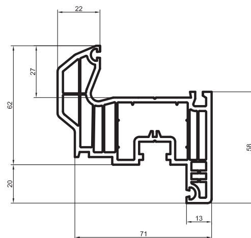
Ablak szárny penta plus 2527
