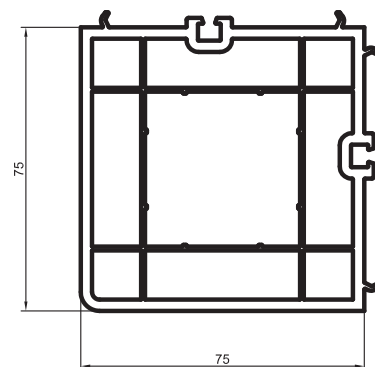
Soroló profil 90° penta 2573
